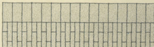
Kantning med kopskifte på fladen
