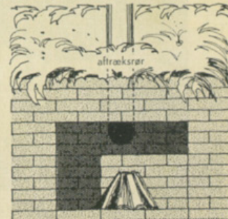
Opstalt
