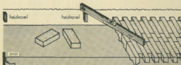
Lægning af klinker ved gange og mindre arealer
