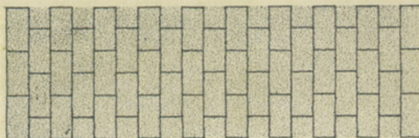
Klinker på fladen, \frac{1}{2} -stens forbandt
