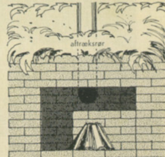
Opstalt Pejs til indbygning i støttetur eller plantekumme mål 1:100, 1:25
