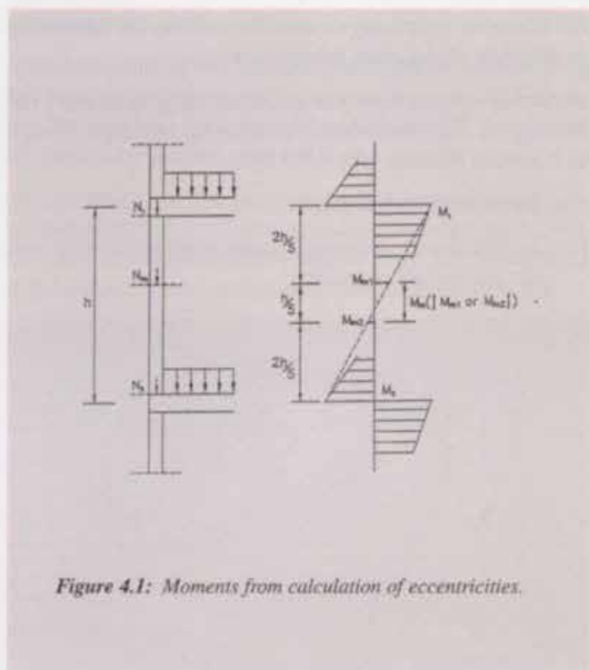
Fig. 1.5 Excentricitetsmomenter efter EC-6.
