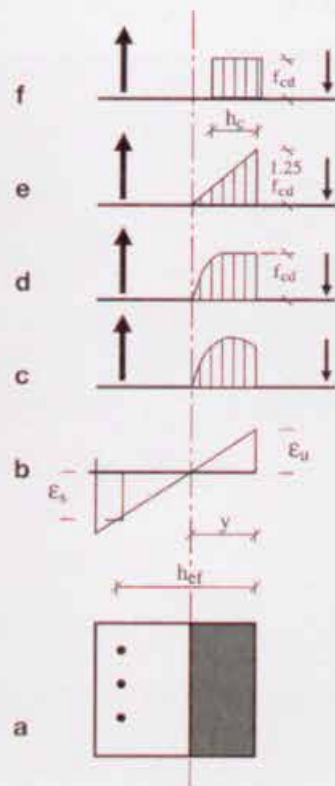
Fig. 2.1 Mulige spændingsfordelinger i momentbelastet væg.
