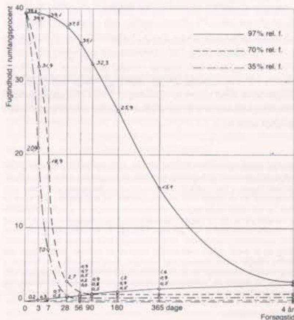
Vandmættet murstens vandafgivelse og tørre murstens vandoptagelse ved lagring i luft med relativ fugtighed 97, 70 og 35%, lufttemperatur 18°C (efter P. Høibø: Der Austrocknung von Baustoffen ).
