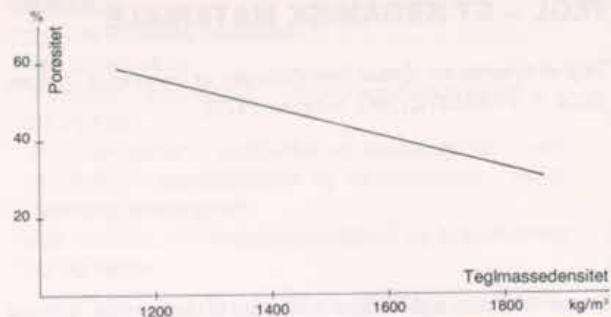
Sammenhæng mellem teglmassedensitet og totalt porevolumen for en teglmasse med densitet 2700 \text{kg/m}^3 for de faste bestanddele.
