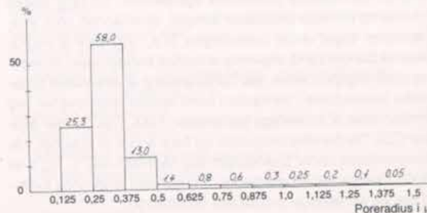
Porene i en tegltagsten fordelt efter vidder.
