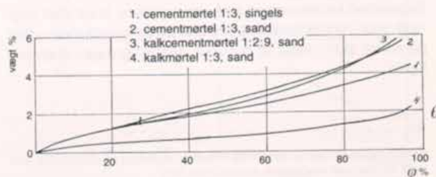
Sorptionsisotermer ved en lufttemperatur på 50°C, middelværdier af absorption og desorption (efter Poul Becher, Varme og Ventilation).
