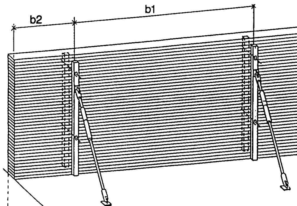
Figur 2. Her er et eksempel på midlertidig afstivning med såkaldte "blådrenge".
