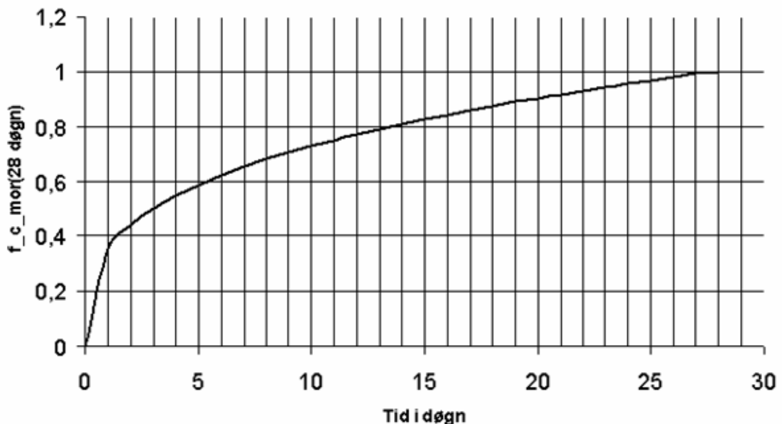
Styrkeudvikling - vedhæftningsstyrken
