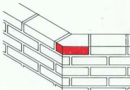
Stumpvinklet udadgående hjørne
