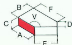
Hjørneste, stumpvinklet 135° indadgående
