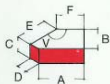
Hjørneste, stumpvinklet 135° udadgående
