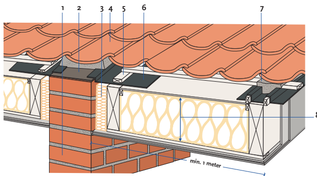
Figur 38. Brandkamserstatning ved brandvæg eller brandsektionsvæg af murværk.
