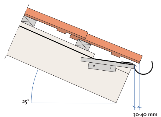
Figur 33. Afslutning ved tagfod med 25° taghældning. Ventilert fuglegitter er ikke vist.
