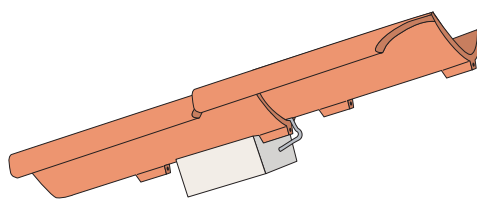
Figur 15. Vingetagsten, krampe. Må kun benyttes som supplement i begrænset omfang, hvor f.eks. JP-bindere eller sidefalsbindere ikke kan anvendes eksempelvis i yderste række over henmurede tagsten.
