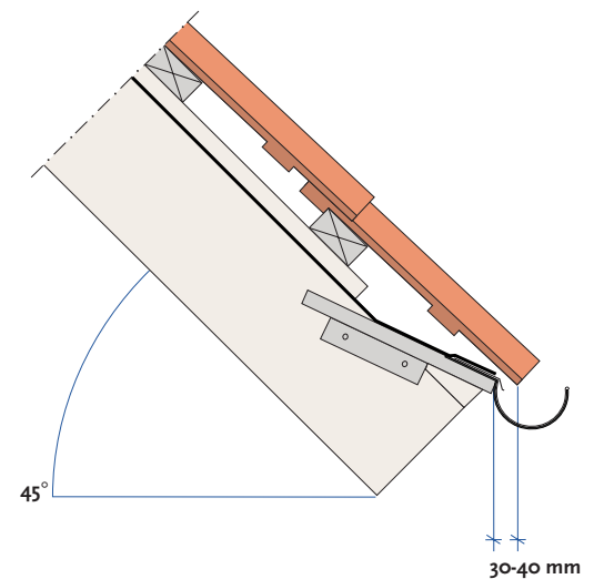
Figur 32. Afslutning ved tagfod med 45° taghældning. Ventilert fuglegitter ikke vist.
