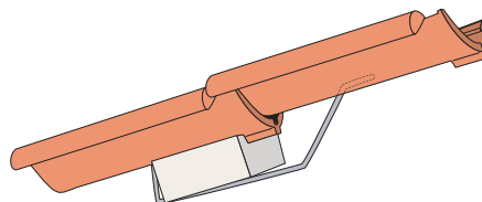
Figur 16. Falstagsten, sidefalsbinder.
