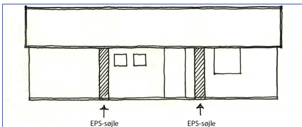
Fig. 3: EPS-søjlerne anbringes på passende steder, typisk midt på et felt mellem dør/vindue. De er ikke synlige i facaden.
