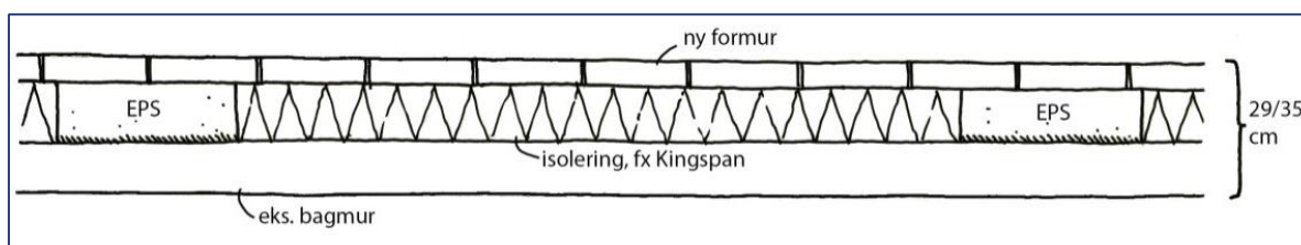
Fig. 4: Vandret snit viser princippet i koncept 1. EPS-søjler afstiver muren; mellem søjlerne er der valgfri isolering, som ikke indgår i det statiske system.
