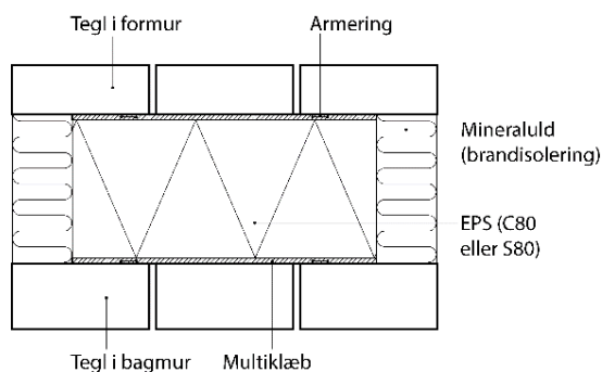
Fig. 1: Vandret snit. Princip for EPS-søjle
