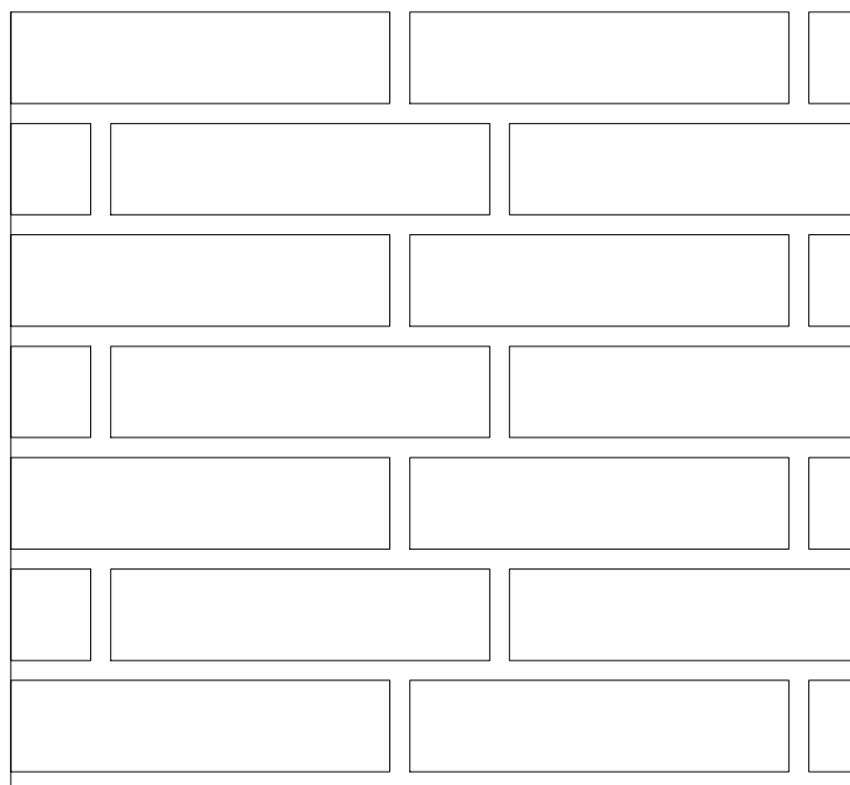
Sten på kant. Kvantstens forbandt
