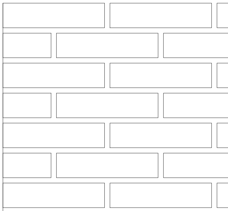
Sten på kant. Halvstens forbandt
