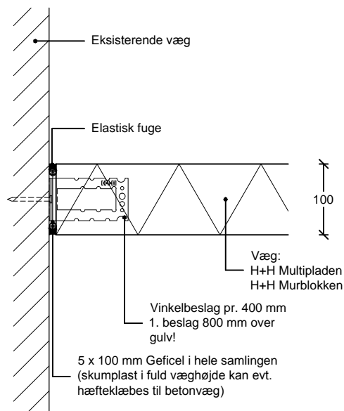
Vandret snit
