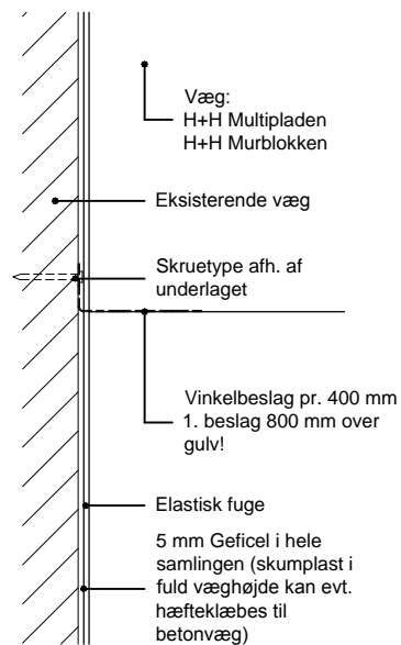
Lodret snit
